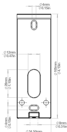
Plaque arrière
