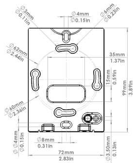
Plaque arrière
