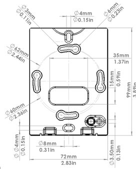
Placa trasera
