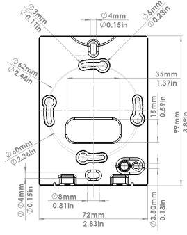
Placa trasera
