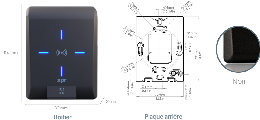
Boîtier
